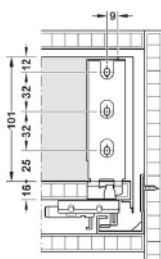
Присадка задней стенки
