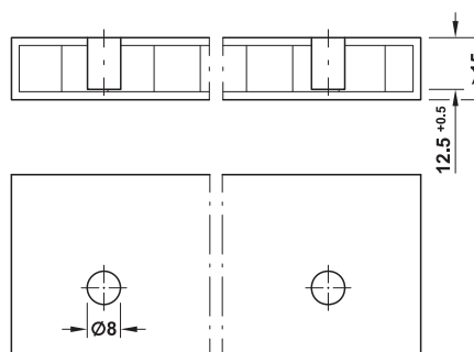
Отверстие на поверхности
