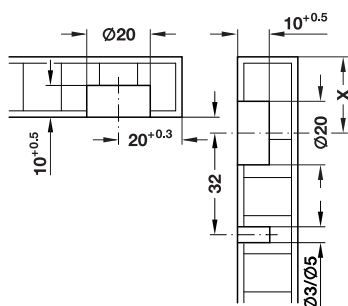
С резьбовым отверстием Размер X = Толщина детали + 4 мм
