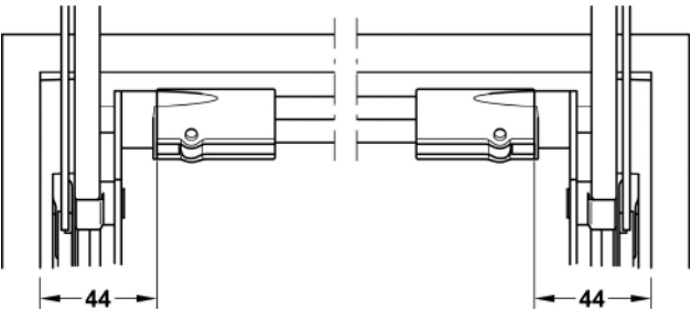
Монтаж синхронизирующей штанги
