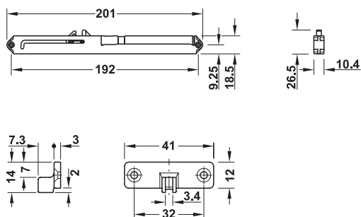
Поводок для деревянного выдвижного ящика
